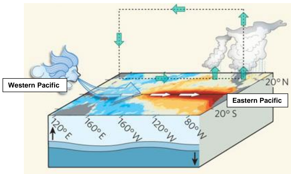
Fig. 8B: El Nino Conditions
